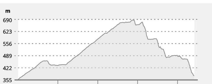
Løypeprofil
